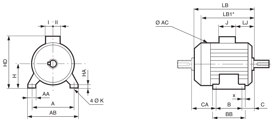
Dimensions principales
