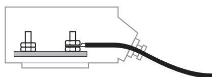
▲ Montage sans cornet
