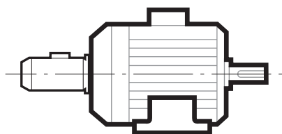
Dynamo tachymétrique*
